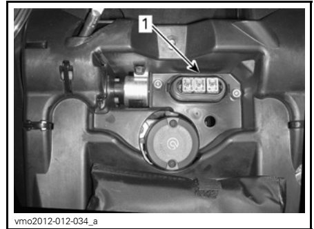
1. Portafusibles trasero
