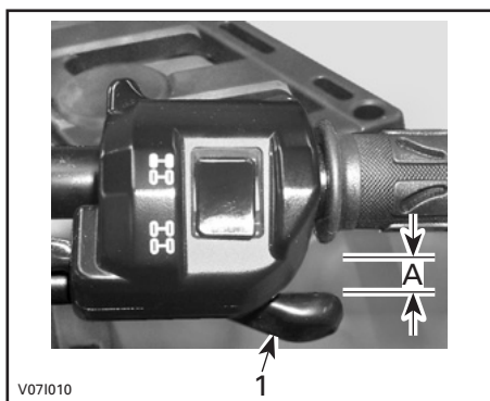
1. Palanca del acelerador A. 3 mm a 6 mm
