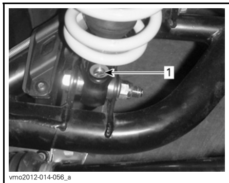
1. Ajustador del rebote (con destornillador plano)
