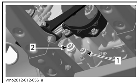
vmo2012-012-056_a TÍPICO - MOTOR 800R 1. Tapón de drenaje 2. Tapón del nivel de aceite
