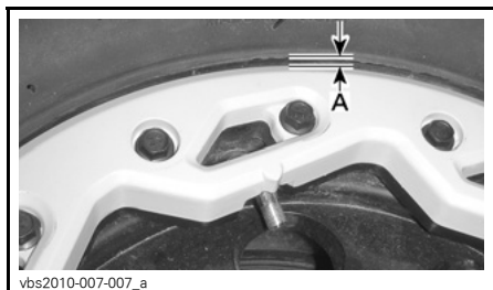
A. Hueco uniforme en el anillo de la abrazadera del sistema de bloqueo de talón
