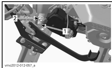
vmo2012-012-057_a TÍPICO - MOTOR 1000 1. Tapón de drenaje 2. Tapón del nivel de aceite
