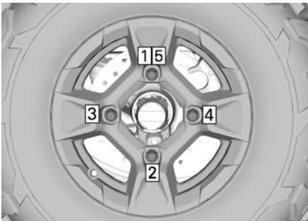
ПОРЯДОК ЗАТЯЖКИ
