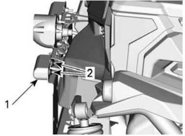
1. Gloeilampkap nummerplaat 2. Borgschroef
