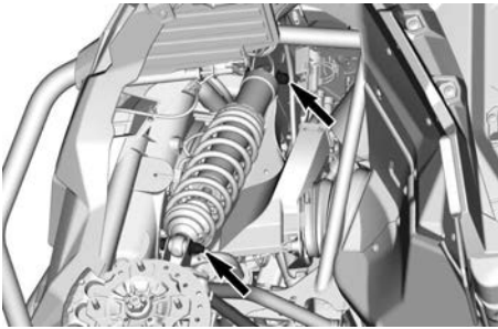
TYPISCH — BEVESTIGINGEN SCHOK-DEMPEER VOOR
