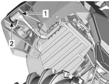
1. Elektrische connector standlicht 2. Borgmoer
