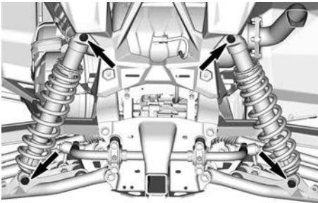
TYPISCH — BEVESTIGINGEN SCHOK-DEMPEER ACHTER
