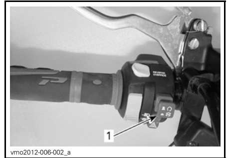
1. Motorstopshakelaar
