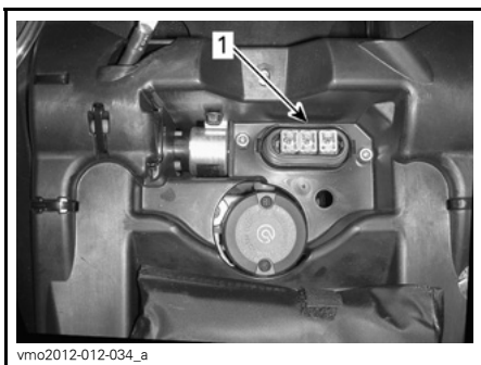
1. Zekeringhouder achteraan
