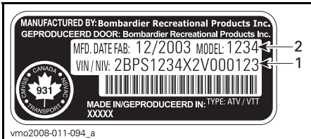
1. V.I.N. (Voertuigidentificatienummer)
