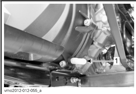
1. CVT-aftapreservoir
