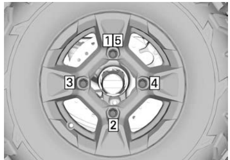
ПОРЯДОК ЗАТЯЖКИ
