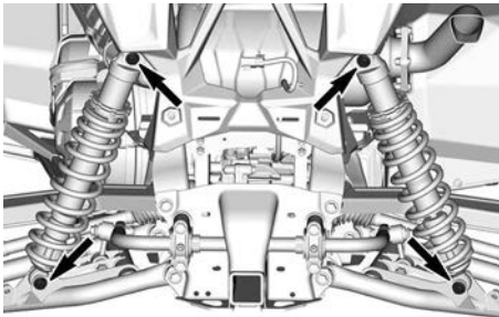
ТИПОВОЙ ВАРИАНТ — КРЕПЕЖНЫЕ ДЕТАЛИ ЗАДНЕГО АМОРТИЗАТОРА
