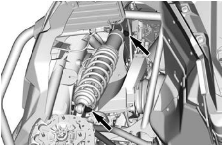
ТИПОВОЙ ВАРИАНТ — КРЕПЕЖНЫЕ ДЕТАЛИ ПЕРЕДНЕГО АМОРТИЗАТОРА
