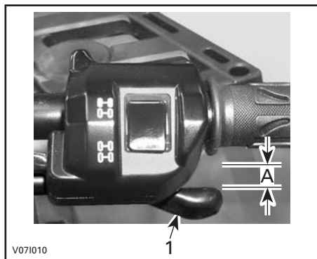
1. Manette d'accélérateur A. 3 mm à 6 mm
