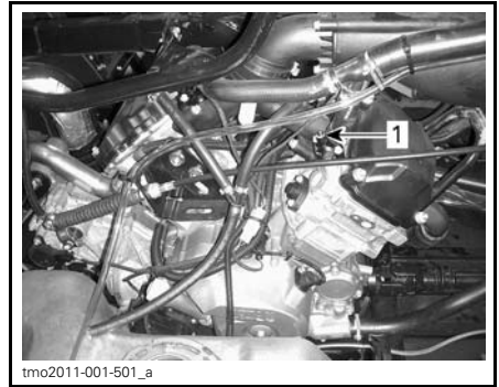
TYPIQUE 1. Vis de purge du cylindre avant
