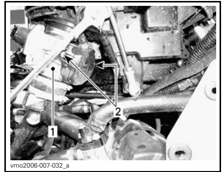
1. Carter de papillon 2. Vis du couvercle latéral
