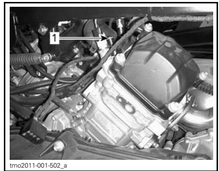
TYPIQUE 1. Vis de purge du cylindre arrière
