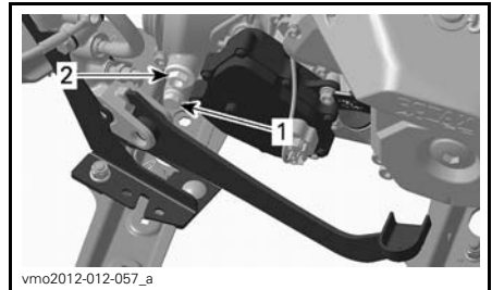
TYPIQUE - MOTEUR 1000
