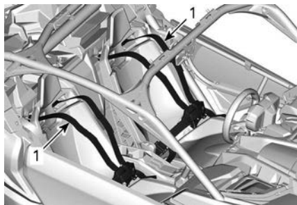
TÍPICO - PIEZAS RETIRADAS PARA MAYOR CLARIDAD
