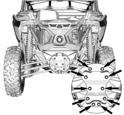
TÍPICO: BARRA ESTABILIZADORA TRASERA
