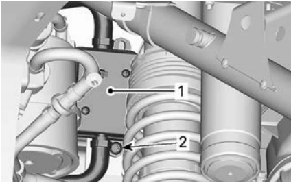
1. Filtre 2. Vis de fixation
