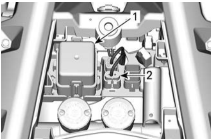
1. Boîte à fusibles avant 2. Fusible DPS
