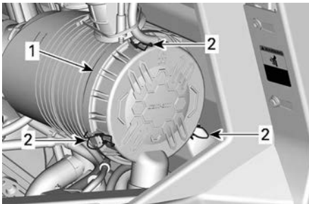
1. Couvercle du filtre à air 2. Verrous
