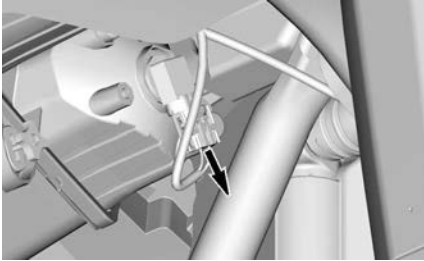
1. Регулировочный винт
