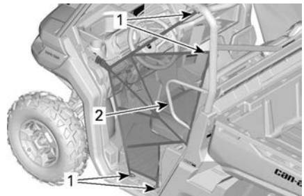
1. Seitennetz-Einstellungsorte 2. Schulterschutz
