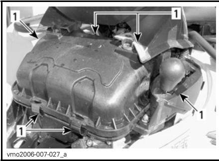
1. Bügel lösen
