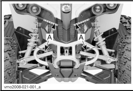
TYPISCH — EINSTELLUNG DER VORSPANNUNG VORN A. Gleiche Länge
