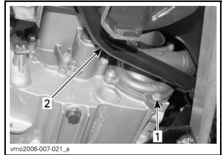
1. Kühlmittelablassschraube 2. Bremspedal
