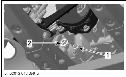
vmo2012-012-056_a TYPISCH - 800R MOTOR
