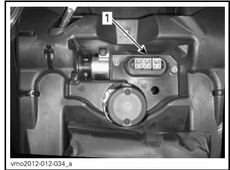
1. Zekeringhouder achteraan
