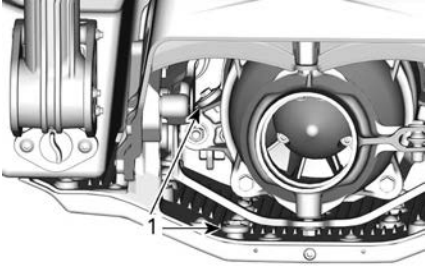
1. Anodi sacrificali
