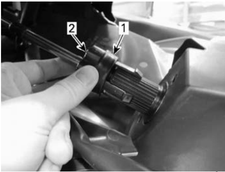
CABLE DE DESENGANCHADO DIRECCIÓN
