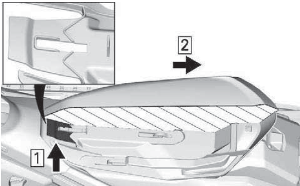
ВИД ПОРОЛОНОВОГО НАПОЛНИТЕЛЯ СИДЕНЬЯ В ПОПЕРЕЧНОМ РАЗРЕЗЕ
