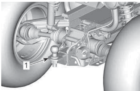
1. Tilhengerfeste
