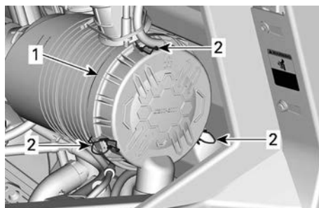
1. Ilmansuodattimen kansi
