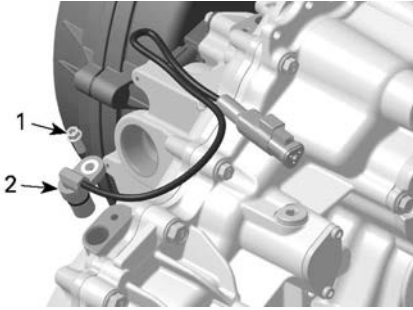
YKSISYLINTERINEN MOOTTORI
