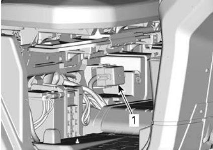
1. Toissijainen takasulakelaatikko
