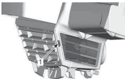
1. Languette de la grille
