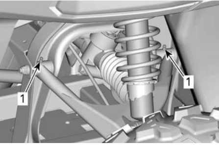
1. Graisseurs du bras de suspension
