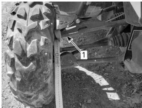
1. Bras de suspension avant supérieur
