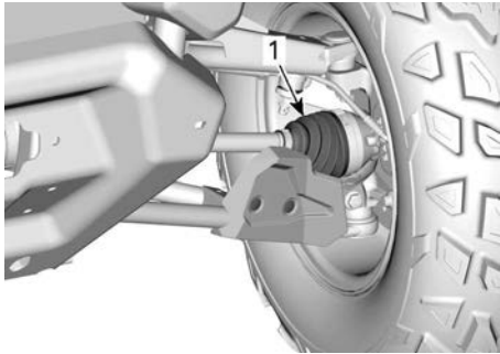
1. Ulommat vetoakselin palkeet
