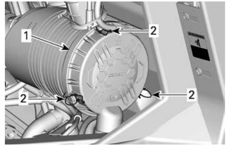
1. Ilmansuodattimen kansi 2. Salvat
