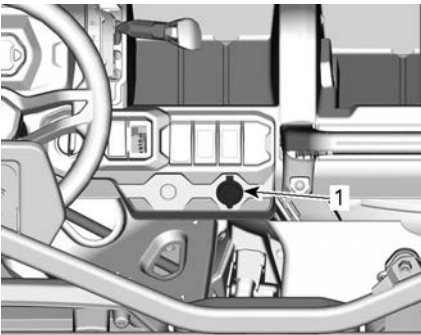
1. 12 V:n pistorasiat
