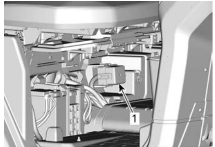
1. Toissijainen takasulakelaatikko
