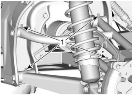
1. Takajousituksen tukivarren rasvanipat
