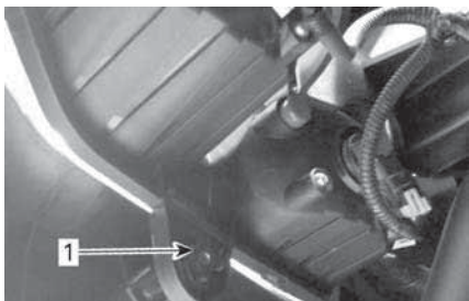
1. Justeringskruv
