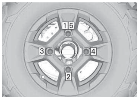
ÅTDRAGNINGSSSEKVEN
