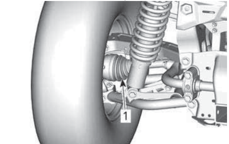
TÍPICO — LADO DE RUEDA TRASERA
