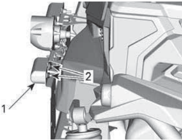
TYPISCH – VORDERRADSEITE
