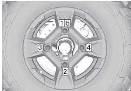
ANZUGSREIHENFOLGE
