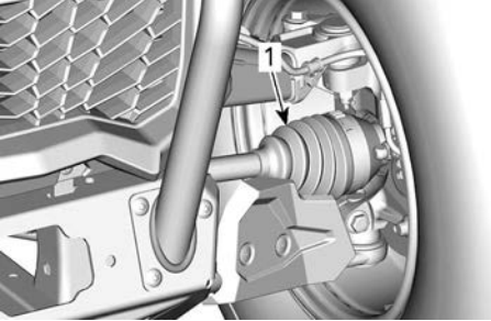
TYPISCH – VORDERRADSEITE
