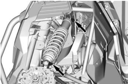
TYPISCH - BEFESTIGUNGSTEILE FÜR VORDEREN STOßDÄMPFER
