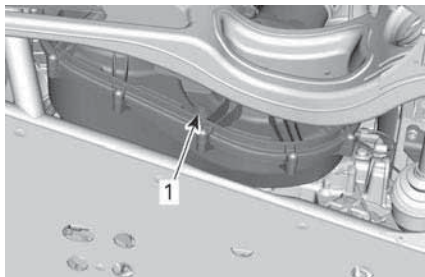
1. Дренаж вариатора
