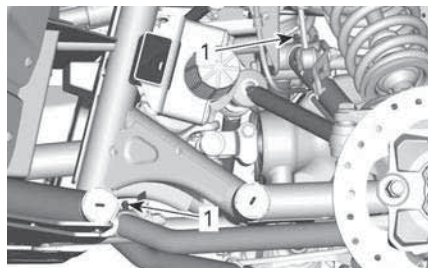
ТИПОВОЙ ВАРИАНТ — ПЕРЕДНЯЯ ПОДВЕСКА
