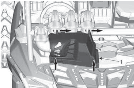
ELEVACIÓN DE LA PARTE TRASERA DE LA TAPA DE ACCESO
