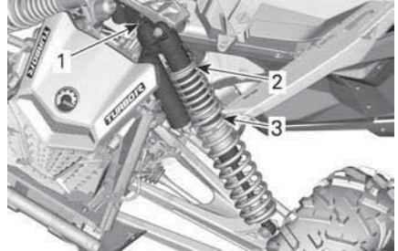
TÍPICO - SIN AMORTIGUACIÓN DE REBOTE - SUSPENSIÓN DELANTERA
