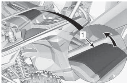
1. 前检修盖
