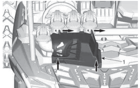
SOLLEVAMENTO DAL RETRO DEL COPERCHIO DI MANUTENZIONE
