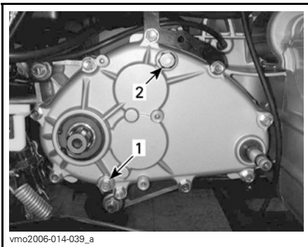
1. Bujão de drenagem do câmbio 2. Bujão de enchimento do câmbio
