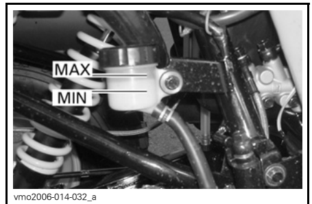
EMBAIXO DO PARA-LAMA TRASEIRO DIREITO
