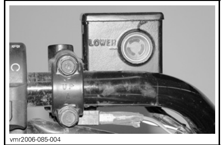
TÍPICO — RESERVATÓRIO DO FLUIDO DO FREIO TRASEIRO ESQUERDO
